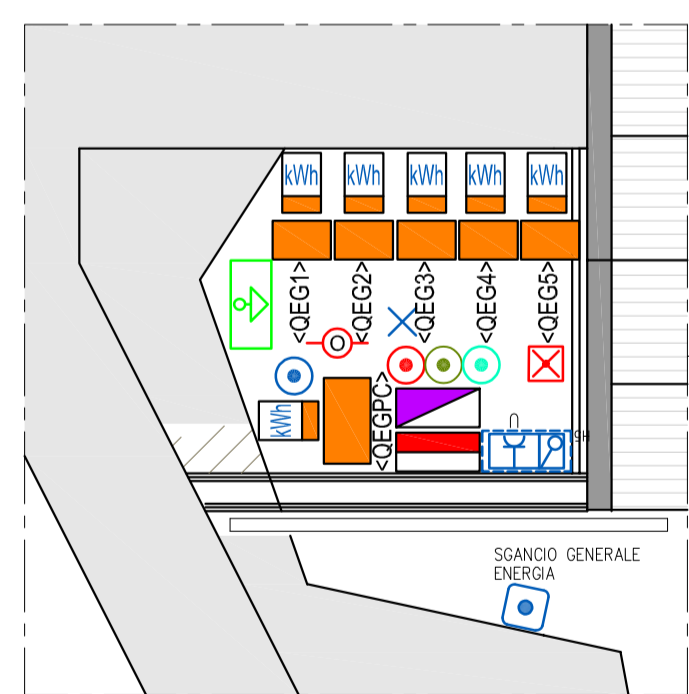
PARTICOLARE SALA QUADRI ELETTRICI Scala 1 : 25
